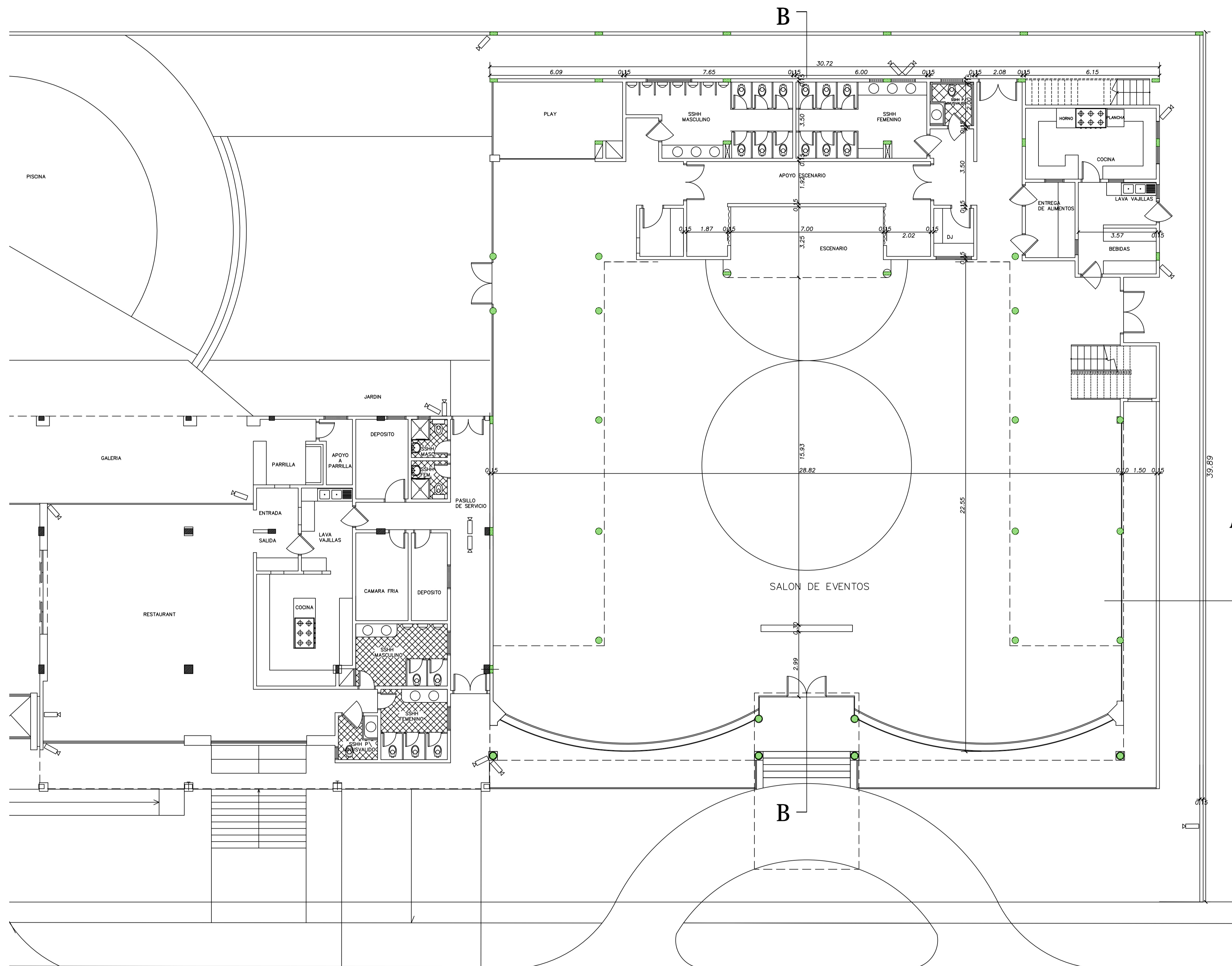
PLANTA BAJA ESC. 1/125
